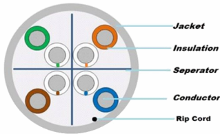
CAT 6 UTP LAN CABLE
